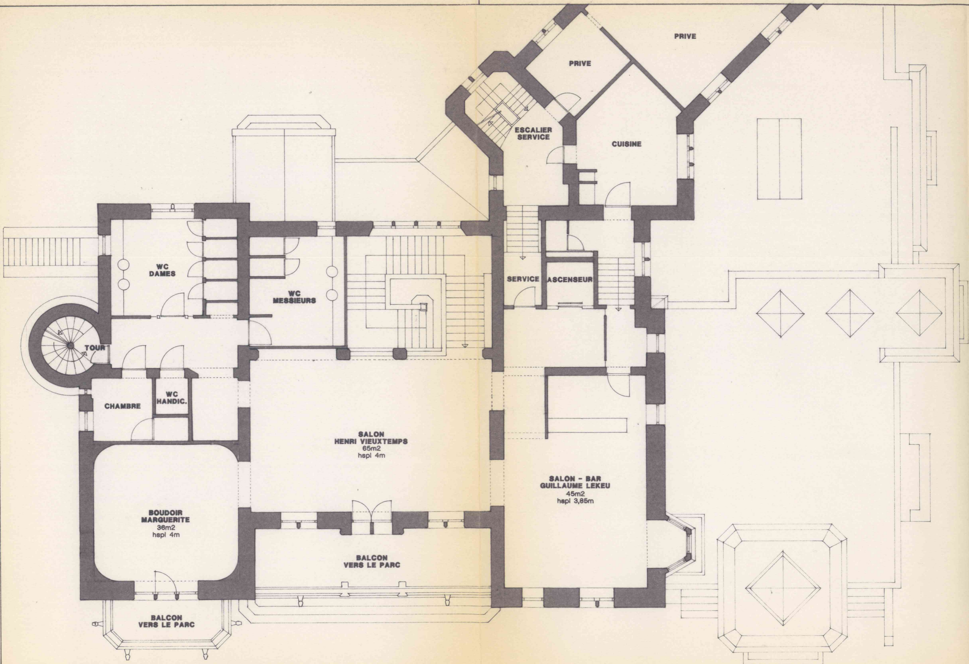
PLAN 1er ETAGE ECH.: 1.100
