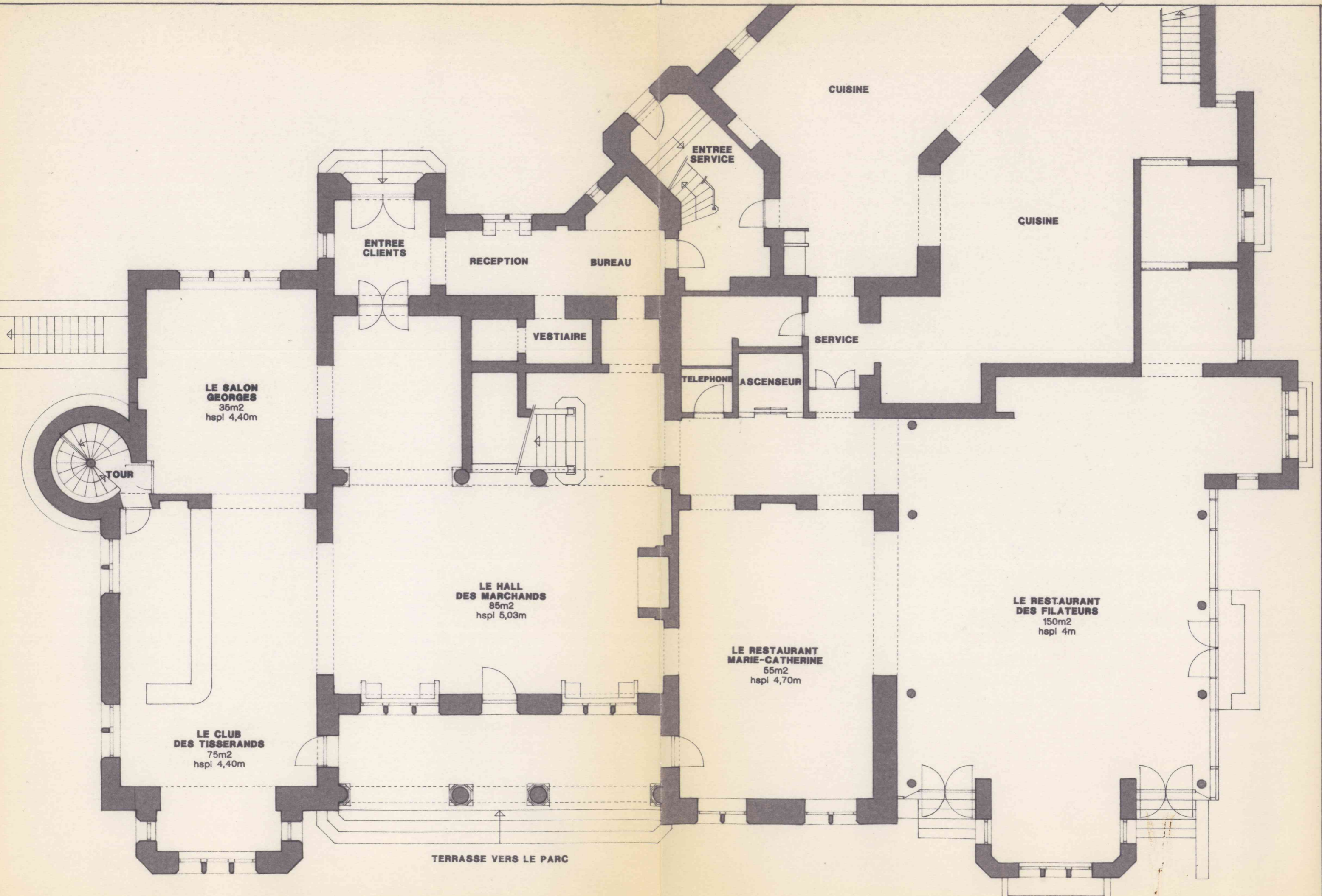
PLAN REZ - DE CHAUSSEE ECH.: 1.100
